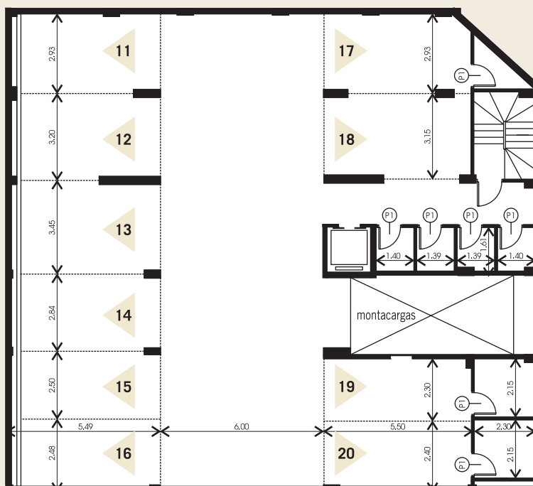
Planta 2º Subsuelo
