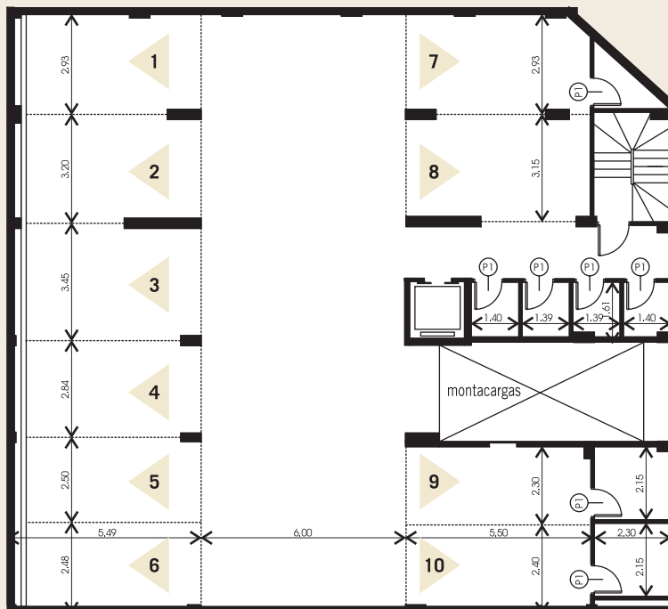
Planta 1º Subsuelo
